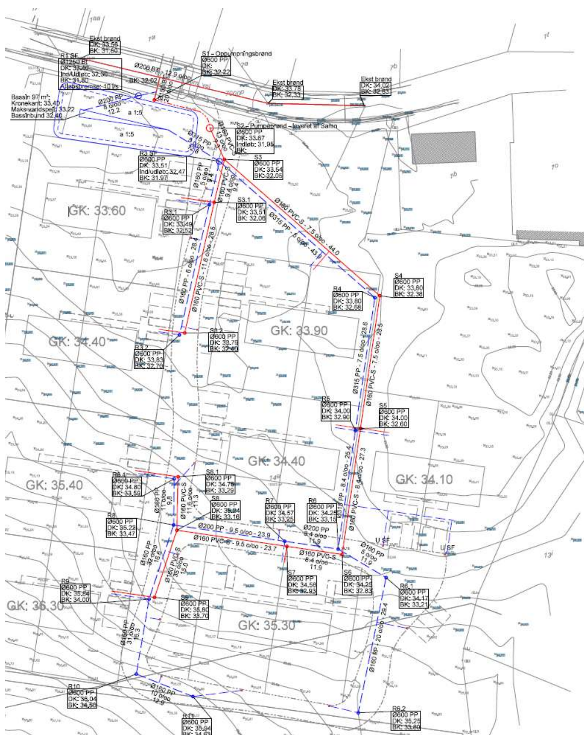
Figur 2: Kloaktegning over regn- og spildevandsledninger, samt tørt bassin og tilslutningspunkt til offentlig fællesledning.
